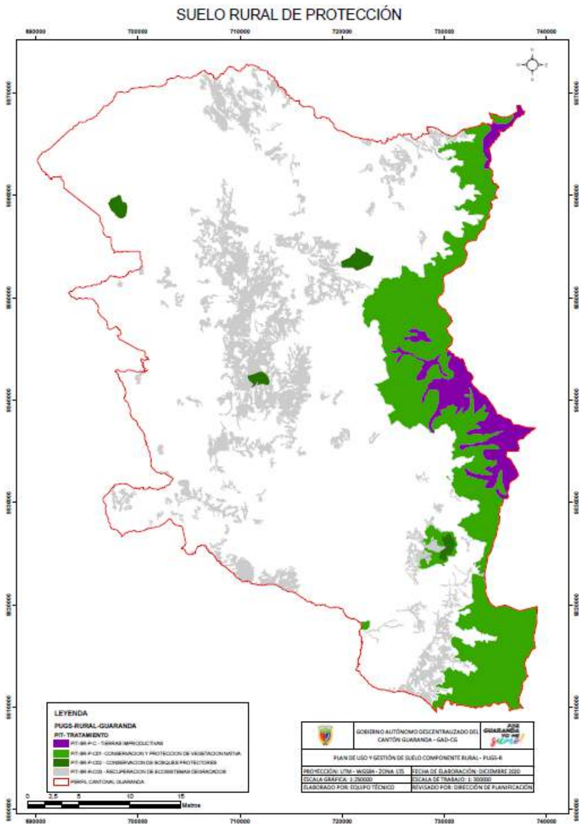
Mapa 48: Suelo rural de protección del cantón Guaranda.
