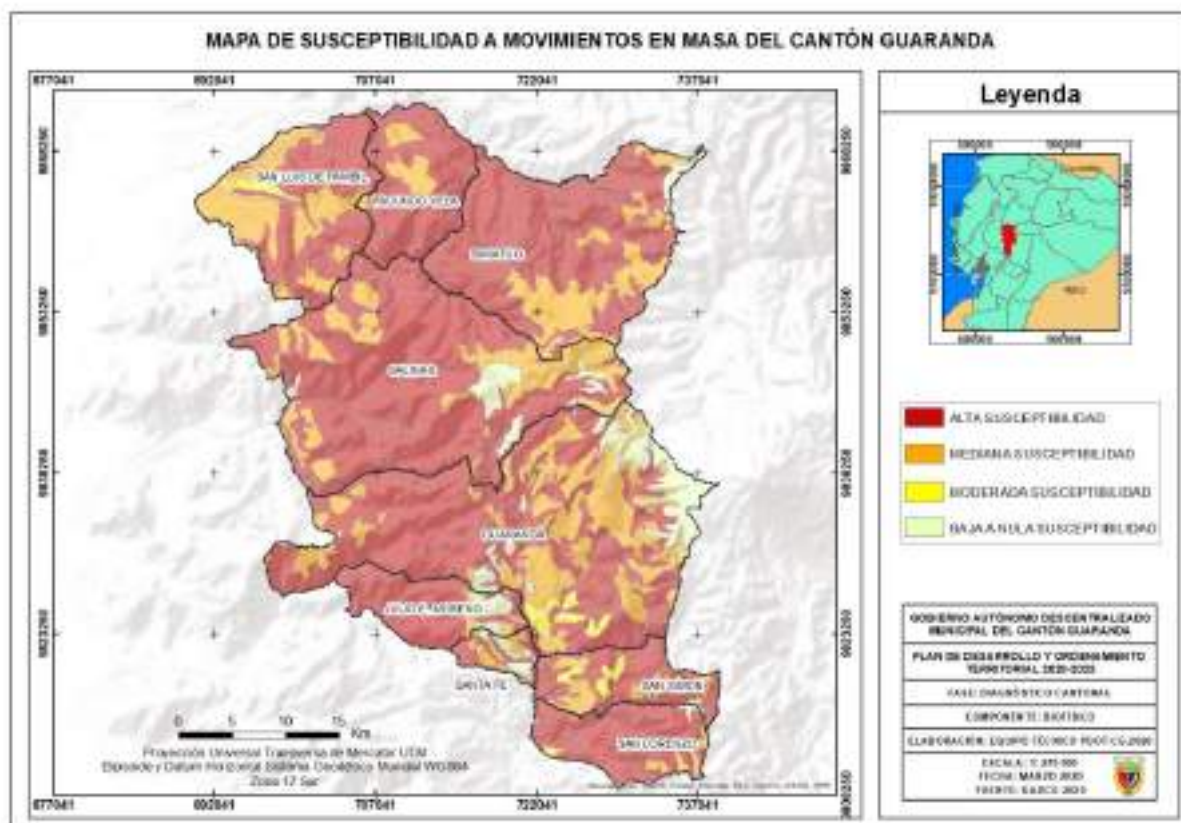
Mapa 15: Susceptibilidad a deslizamientos en el cantón Guaranda.
