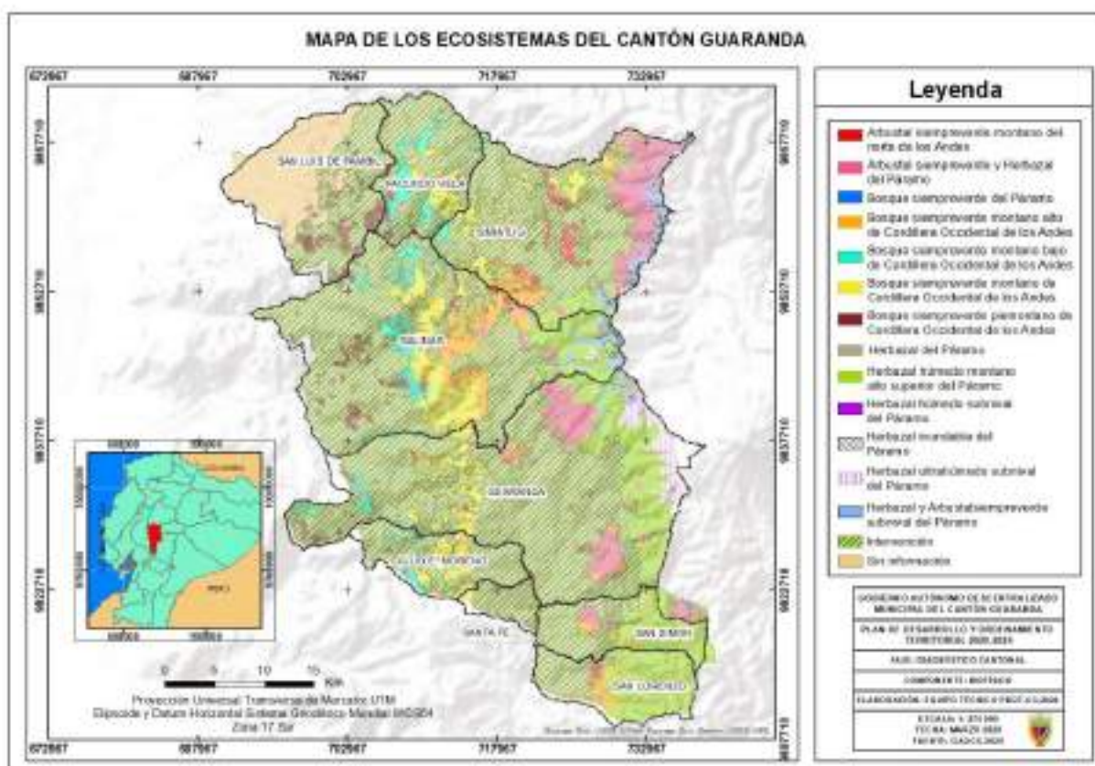
Mapa 14: Ecosistemas del cantón Guaranda.
