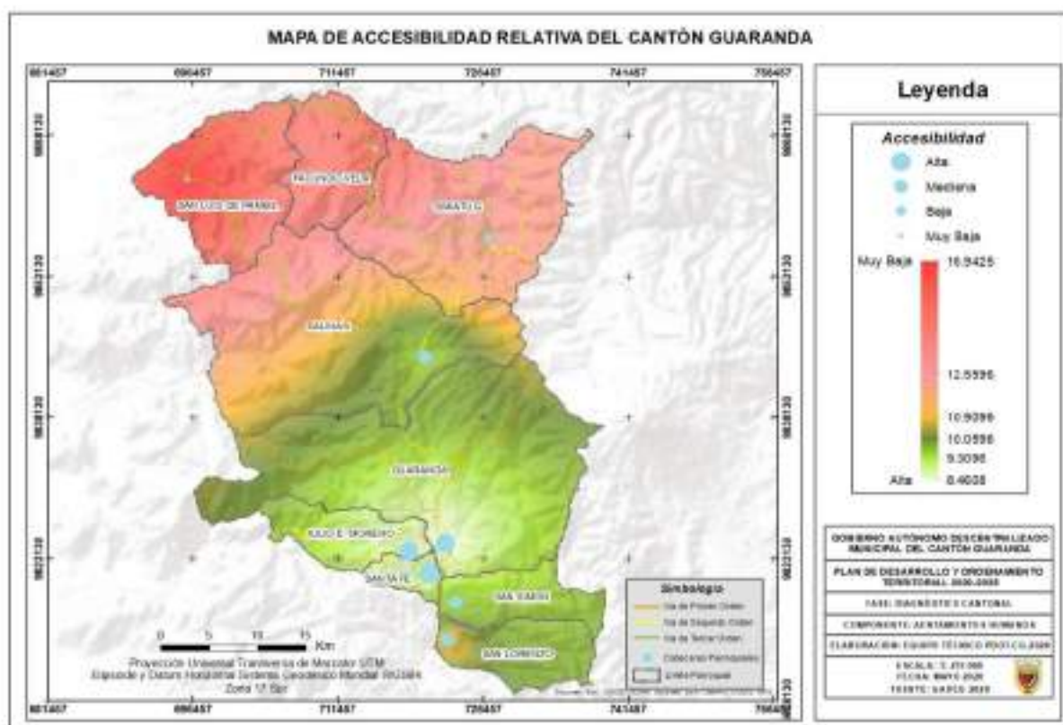
Mapa 32: Accesibilidad relativa del cantón Guaranda.
