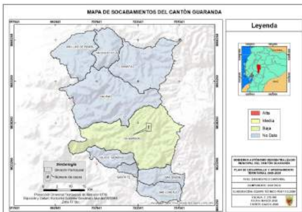
Mapa 40: Sectores expuestos a socavamientos en el cantón Guaranda.
