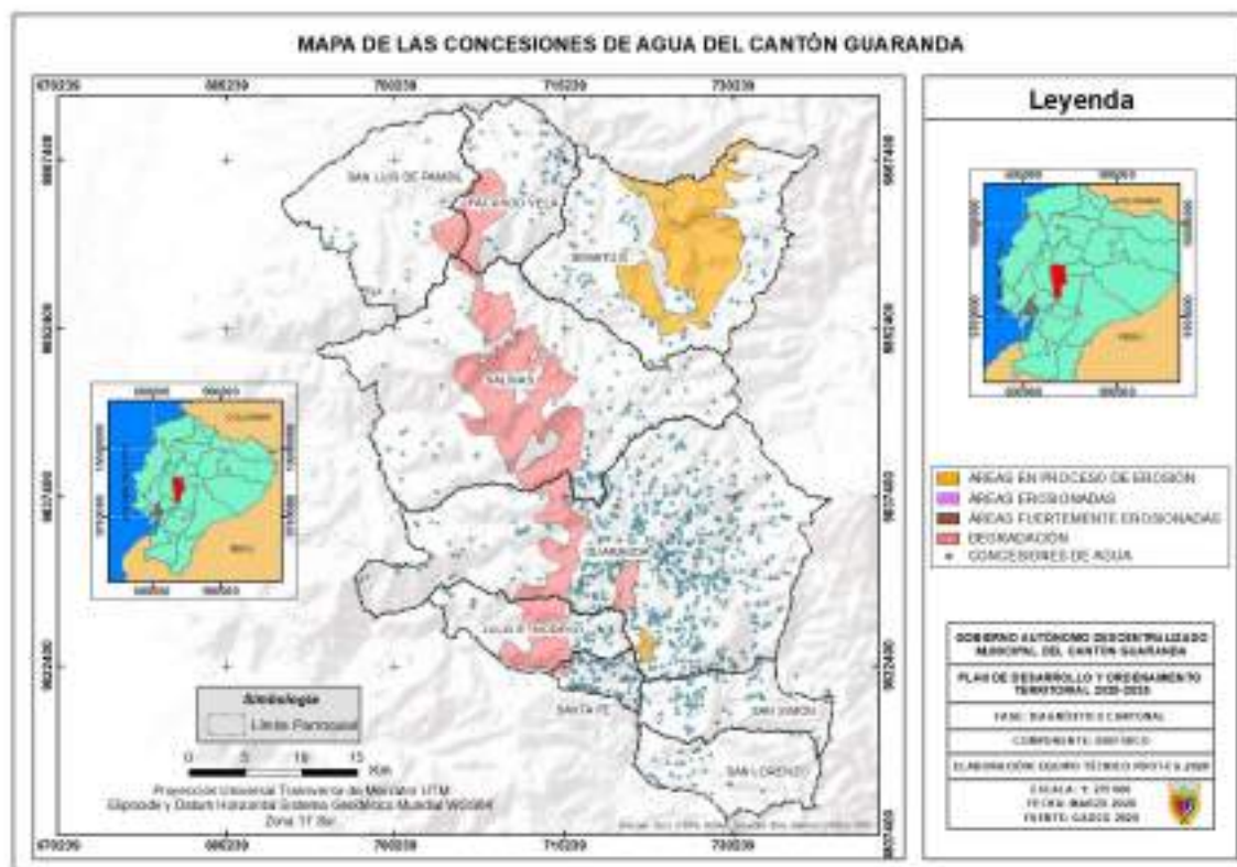
Mapa 1: Las concesiones de agua del cantón Guaranda.
