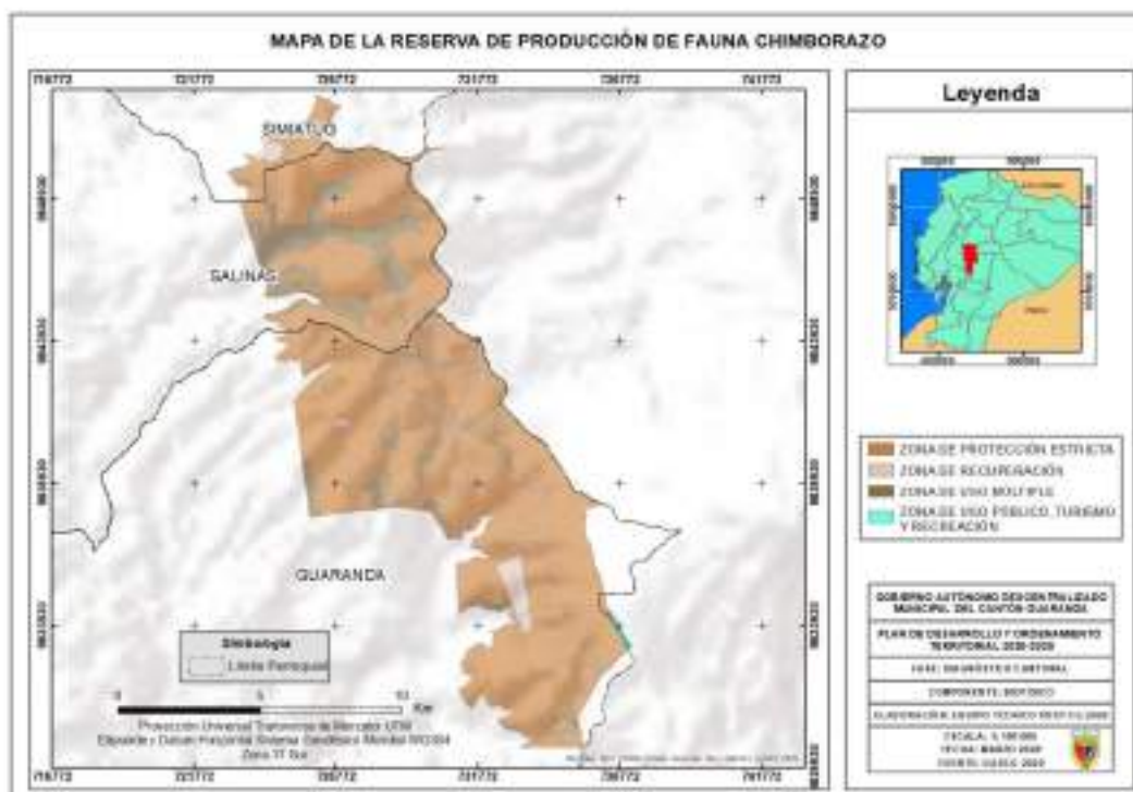
Mapa 3: Reserva de producción de fauna Chimborazo.
