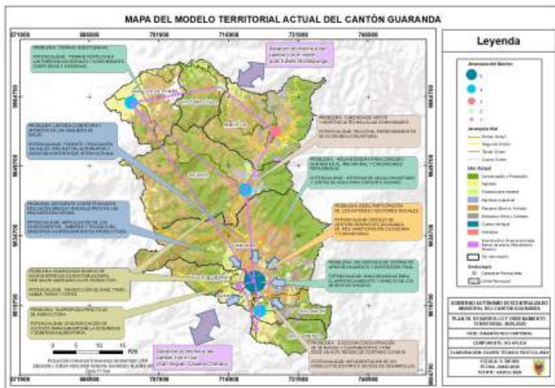
Mapa 44: Modelo territorial actual del cantón Guaranda.
