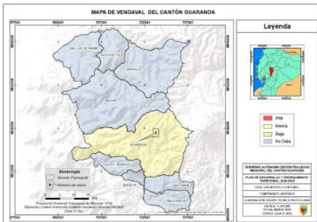
Mapa 41: Sectores expuestos a vendaval en el cantón Guaranda.
