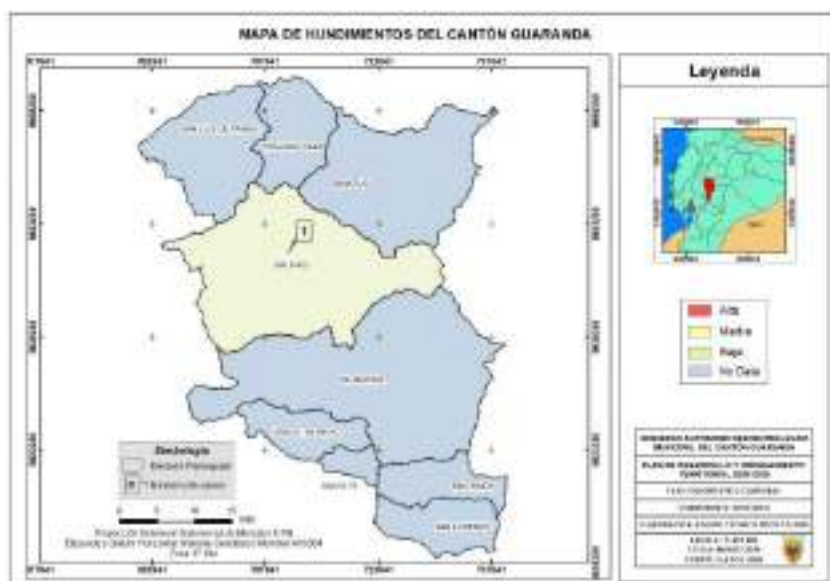
Mapa 37: Sectores expuesto a hundimientos en el cantón Guaranda.
