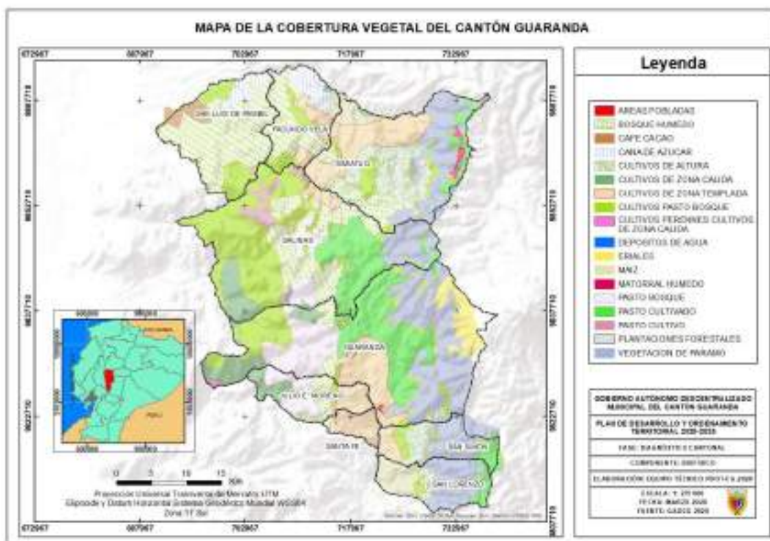
Mapa 12: Cobertura vegetal del cantón Guaranda.
