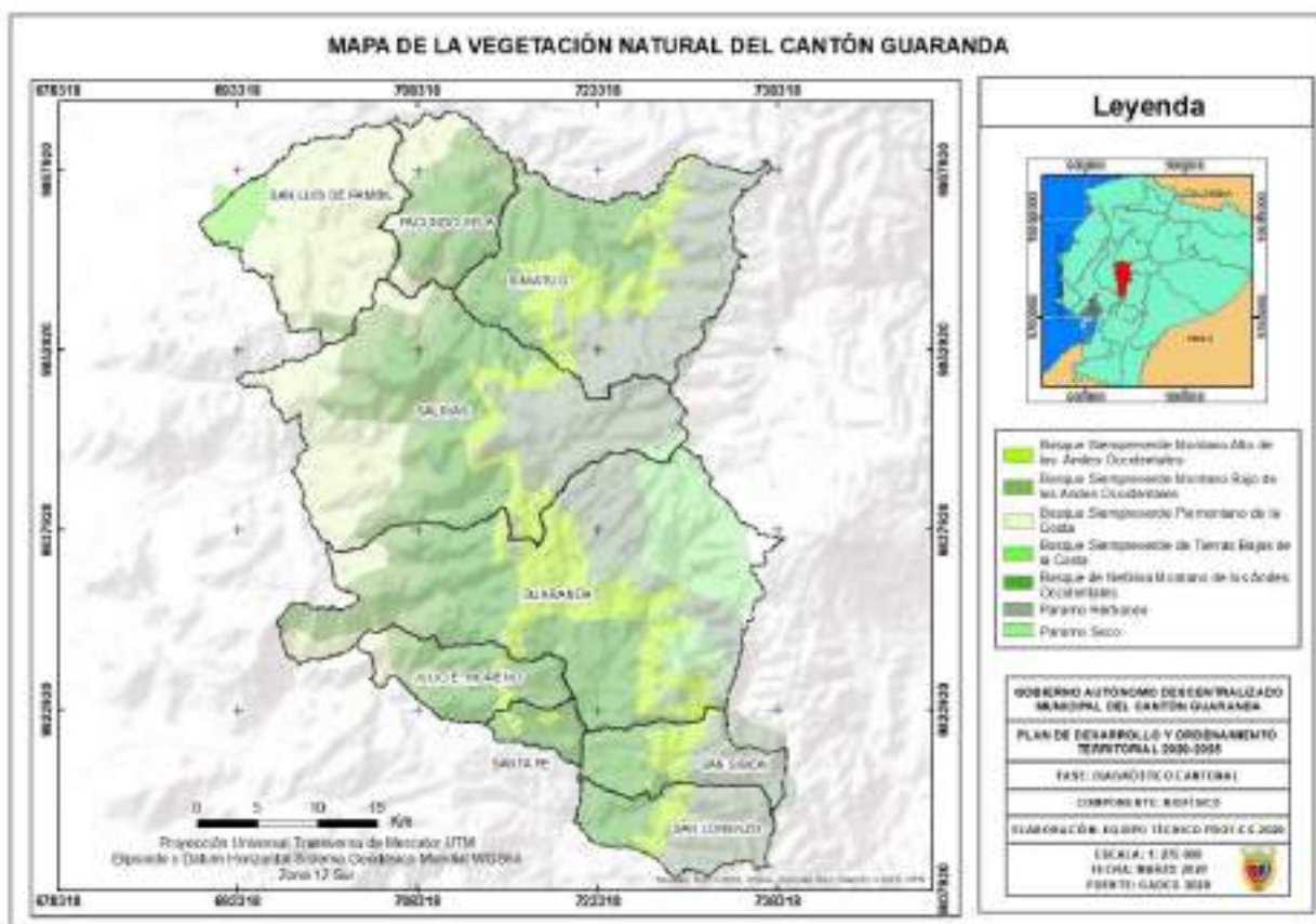
Mapa 13: Vegetación natural del cantón Guaranda.
