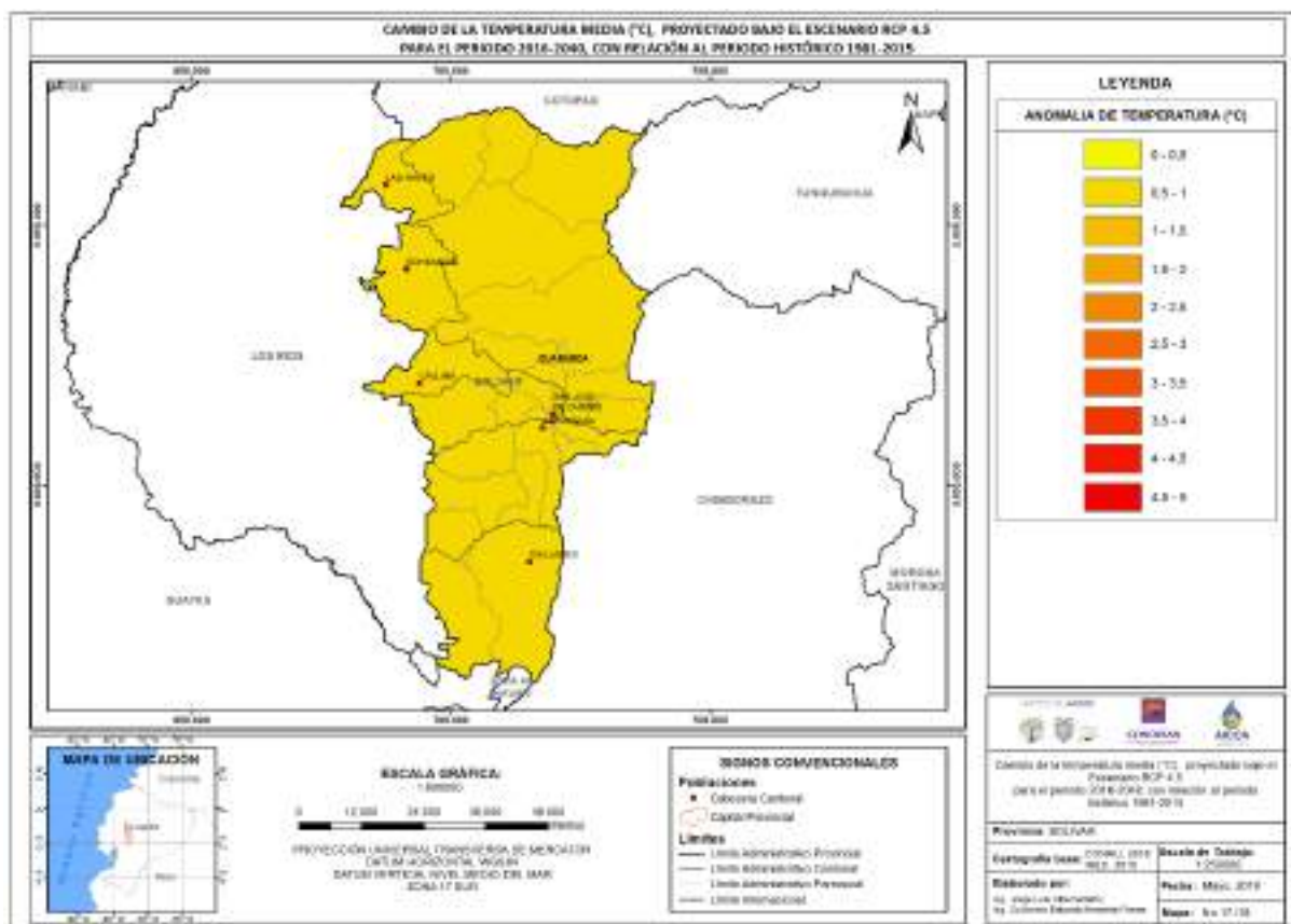
Mapa 6: Aumento de temperatura en la provincia Bolívar.
