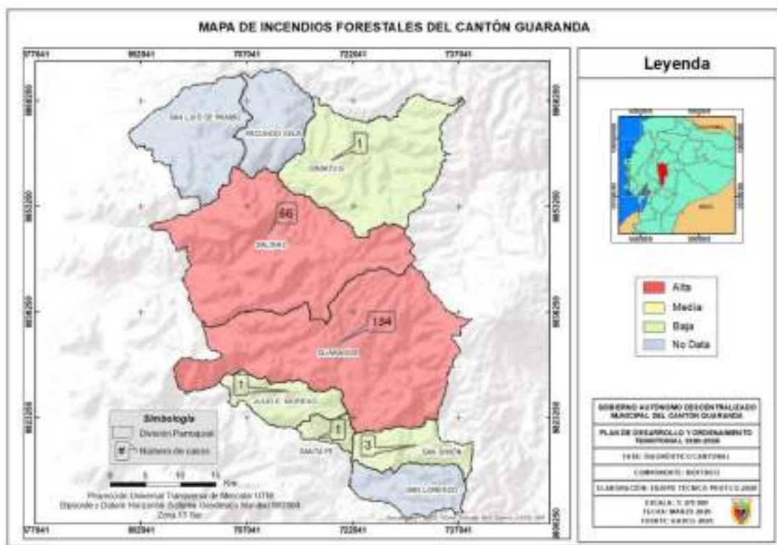
Mapa 39: Sectores expuestos a incendios forestales en el cantón Guaranda.
