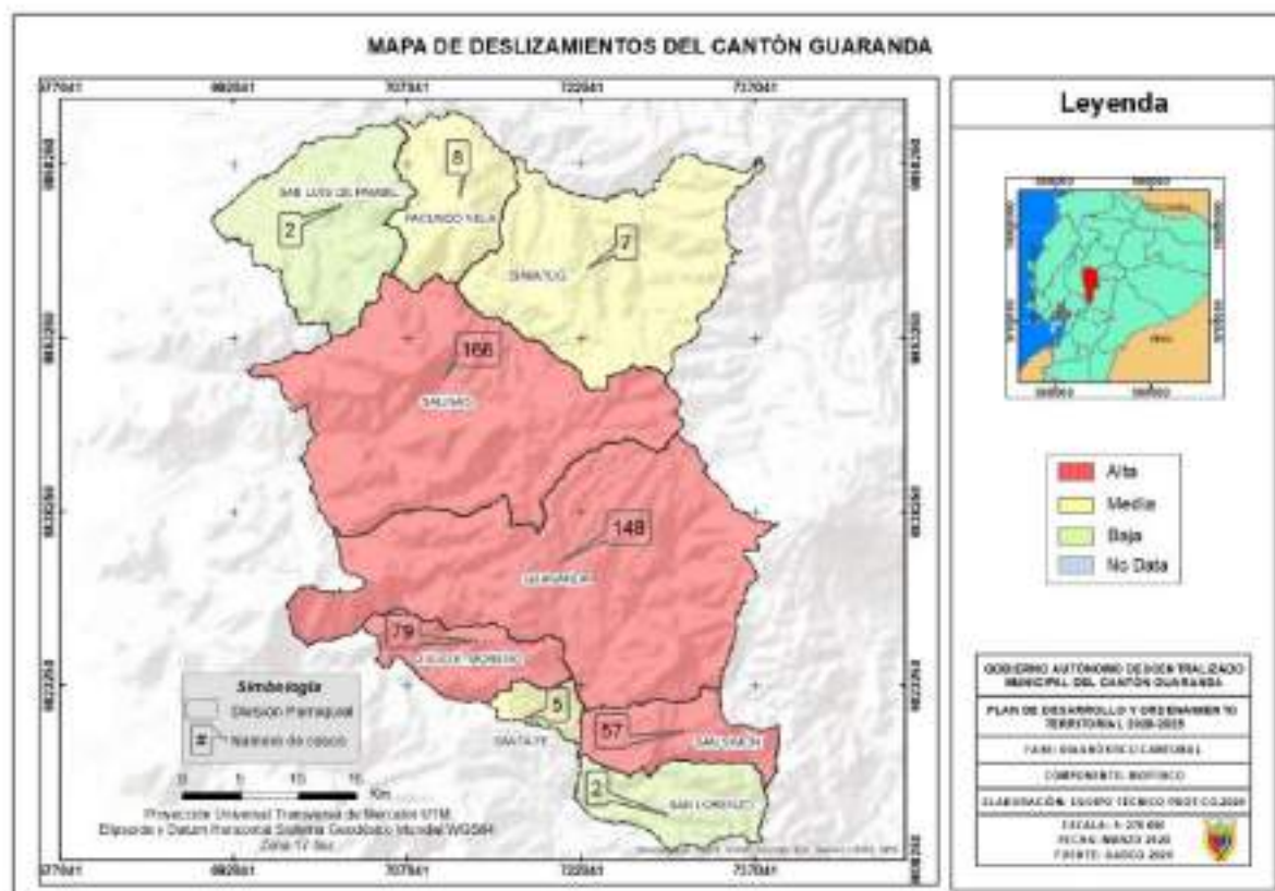
Mapa 36: Sectores expuesto a deslizamientos en el cantón Guaranda.
