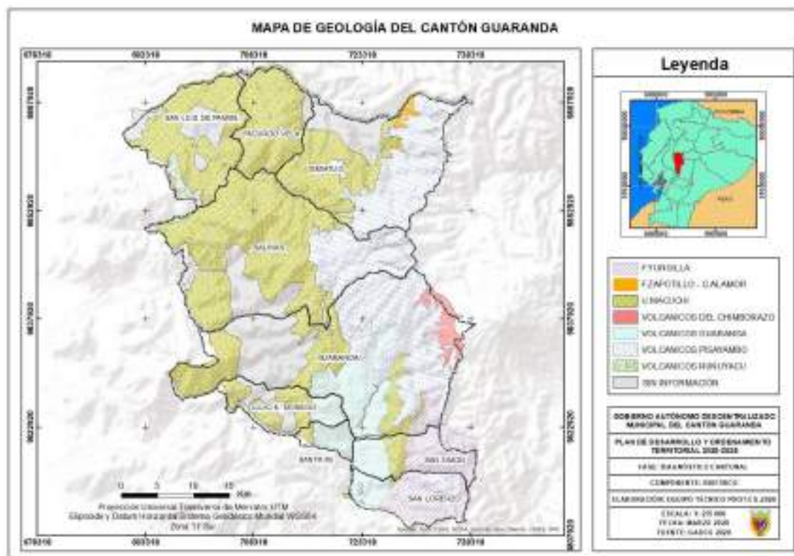
Mapa 8: Geología del cantón Guaranda.
