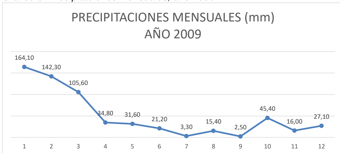
Gráfico 3: Precipitaciones mensuales, año 2009.
