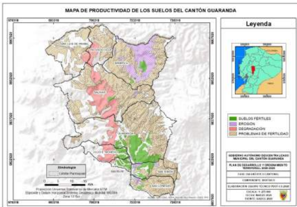
Mapa 10: Productividad de suelos del cantón Guaranda.
