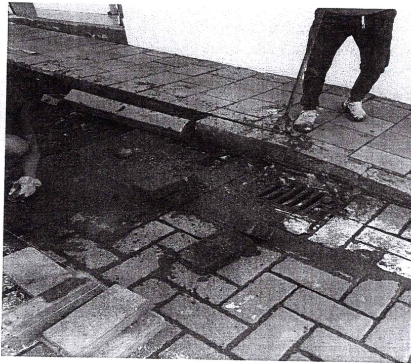
remocion de bordillos sector sumidero actual
