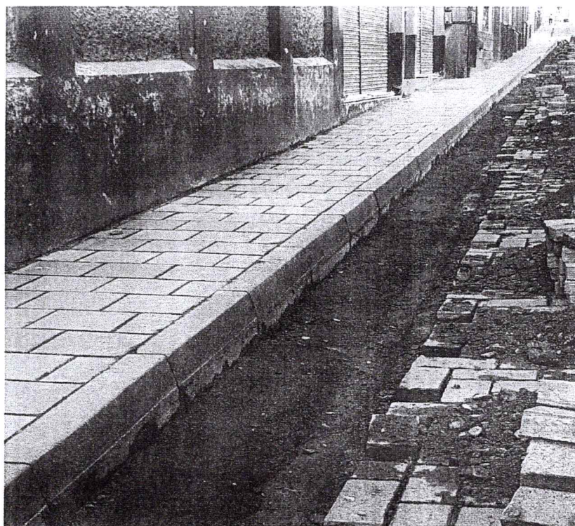
excavacion para bordillo y ensanche de acera
