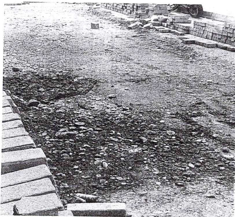
VISTA DE RELLENO COMPACTADO CON LASTRE
