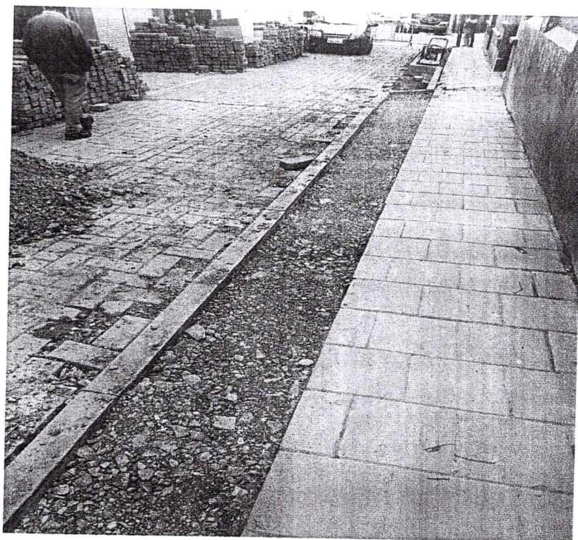
otra vista de relleno compactado con lastre
