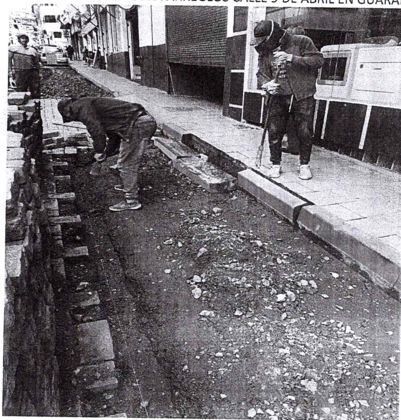
FOTOS OBRA ARREGLOS CALLE 9 DE ABRIL EN GUARANDA
