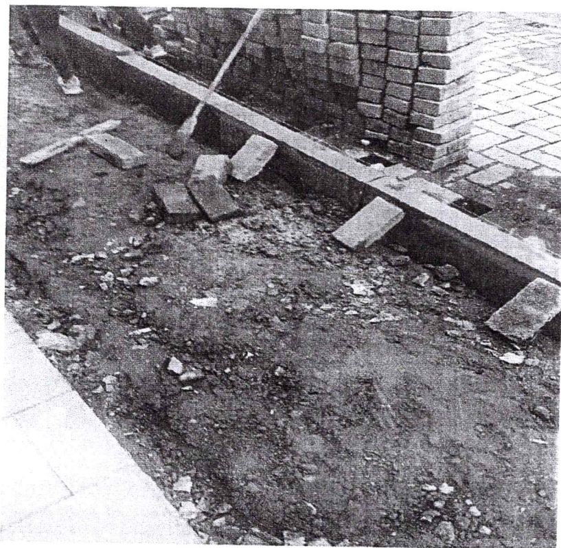
nivelacion y colocacion bordillos en la nueva posicion del ensanche de la acera
