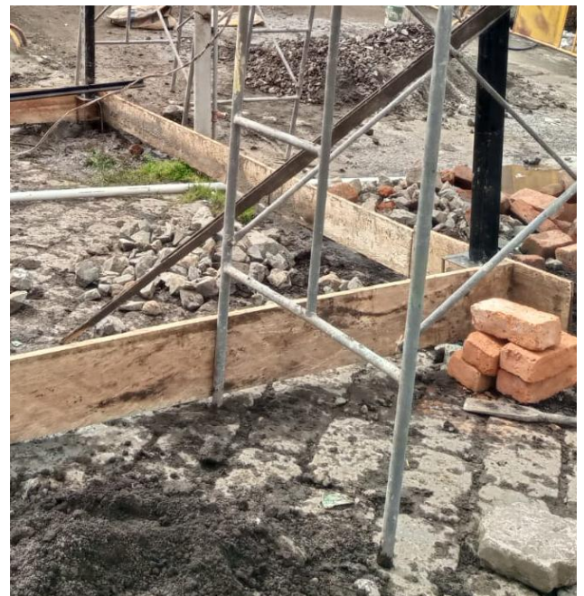
ENCOFRADO PARA CADENAS
