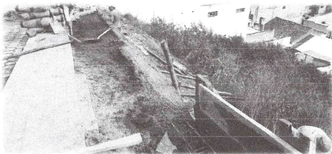
FUNDICIÓN DE MURO, ENCOFRADO, RELLENO Y COLOCACIÓN DE ADOQUIN ORNAMENTAL
