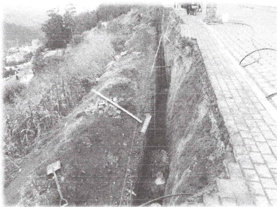
EXCAVACIONES Y FUNDICION DE PLINTOS
